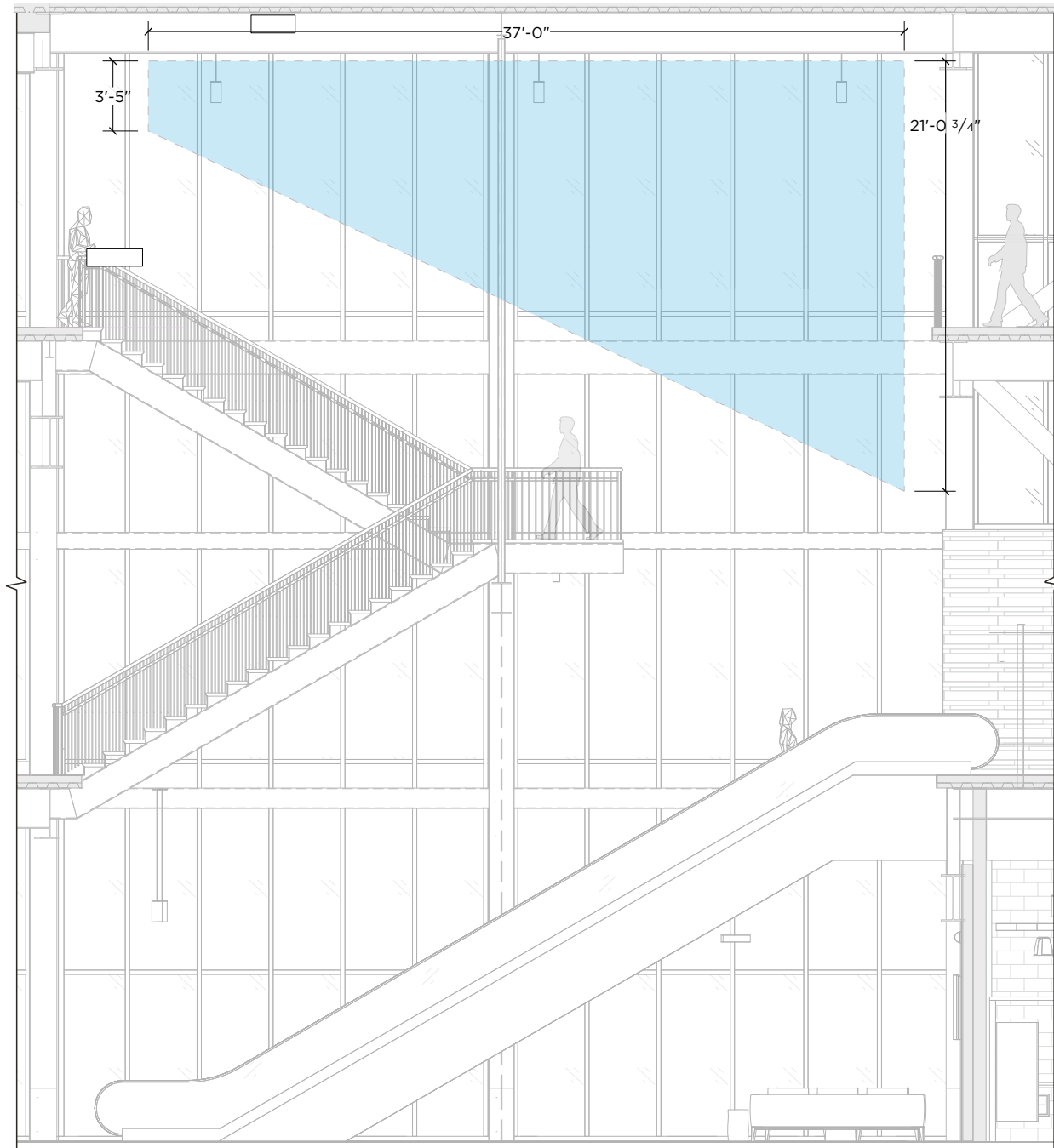
A CONTEXT ELEVATION SCALE: 1/8"=1'-0"
